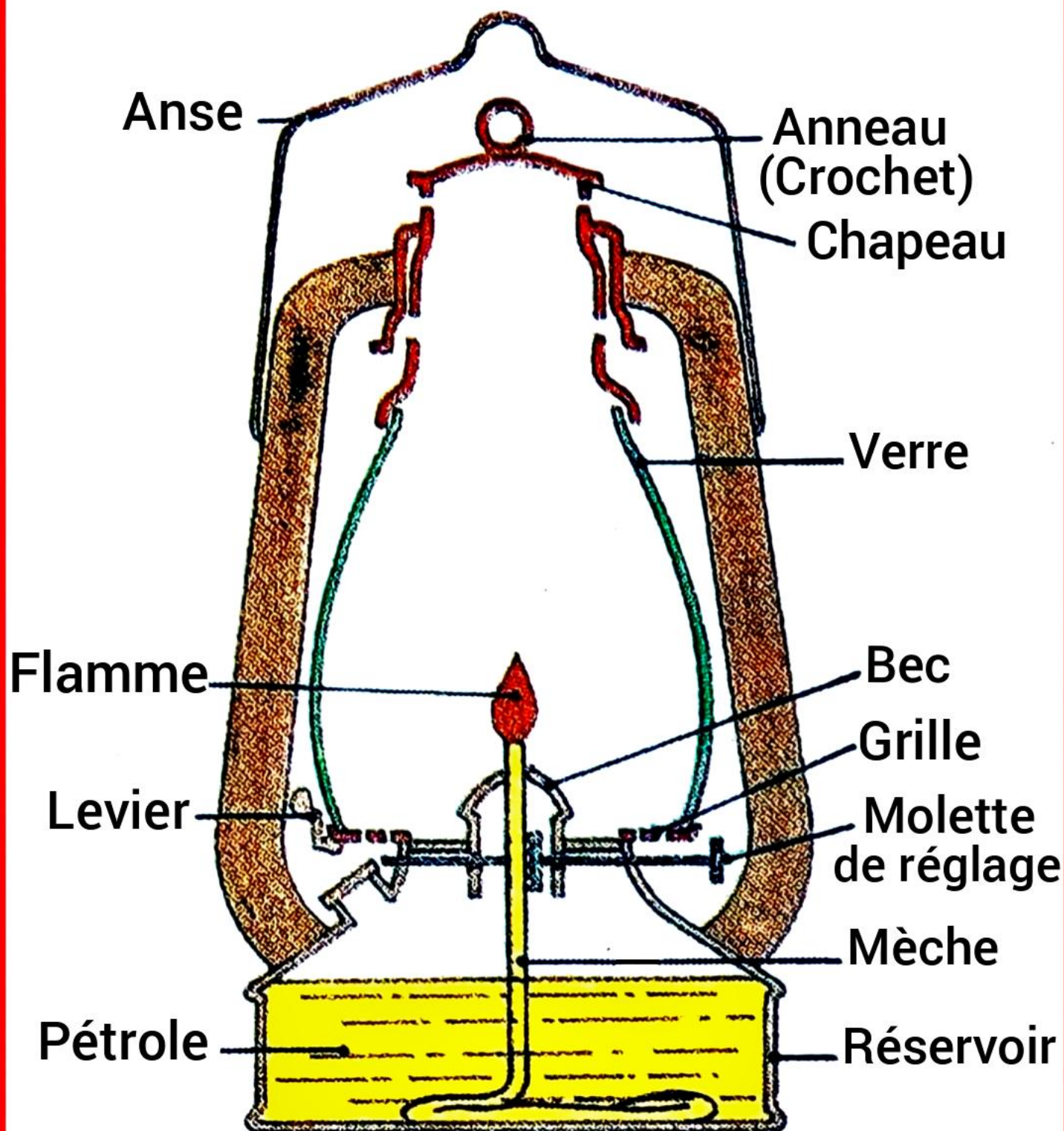
Croquis d'une lampe-tempête
